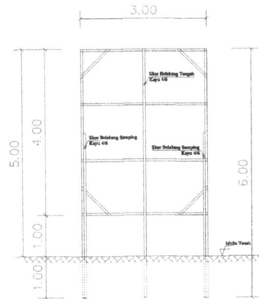
TAMPAK BELAKANG
