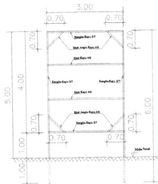
TAMPAK DEPAN
