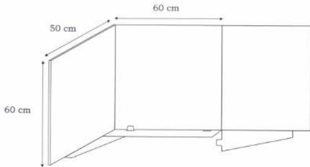
bilik pemungutan tampak terangkai
