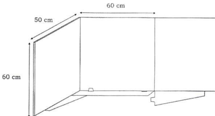
bilik pemungutan tampak terangkai
